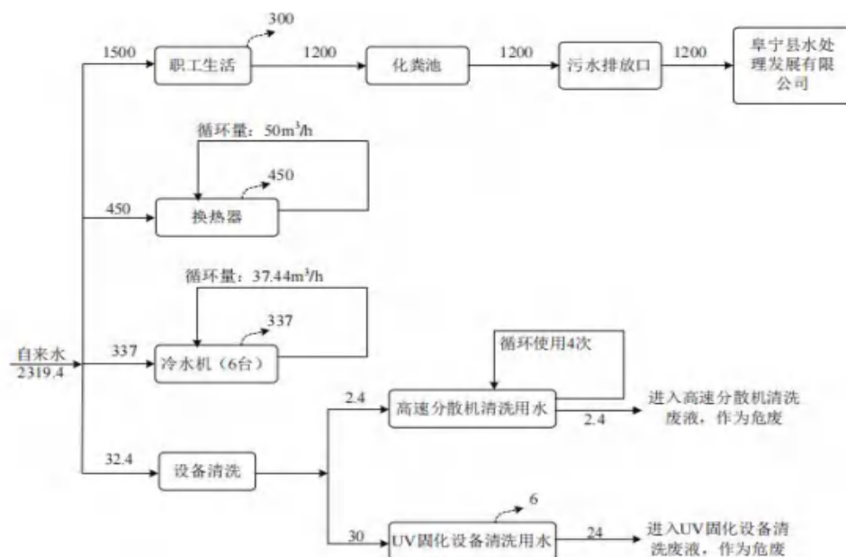
图 3.4 新建项目水量平衡图（单位：m³/a）
